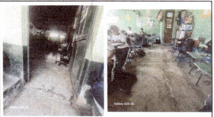
Foto 4: PISO: sustitución de piso ceramico. 4 aulas y pasillo.
